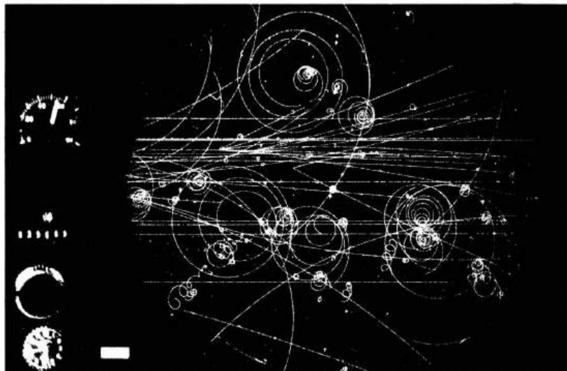
В зависимости от размера и заряда различные субатомные частицы проделывают разные виражи и прокладывают разные спиралевидные траектории, проносясь через пузырьковую камеру. Следы на этой иллюстрации — линии из мельчайших пузырьков, сфотографированных в холодной бане из жидкого водорода (иллюстрация любезно предоставлена ЦЕРН)
